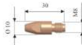
Ddifuzor gaz 501w
